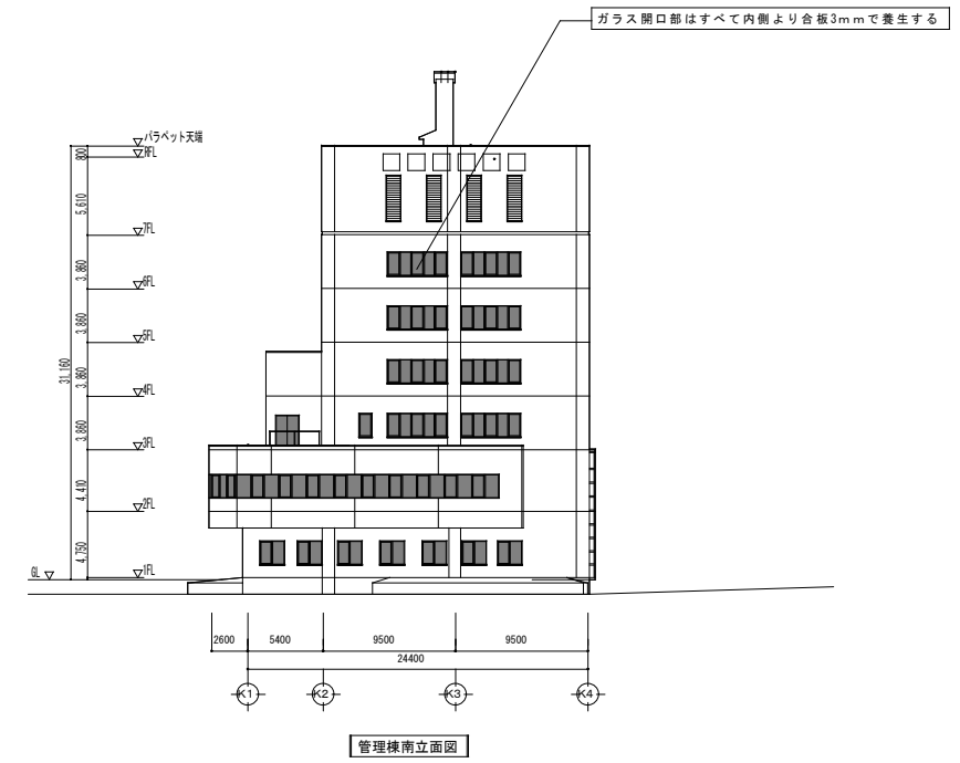
管理棟南立面図
