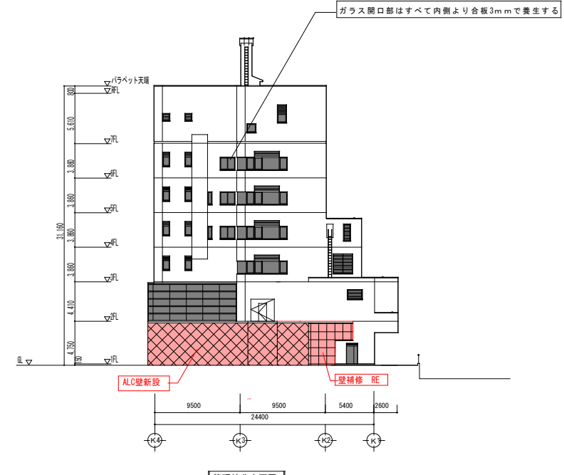
管理棟北立面図
