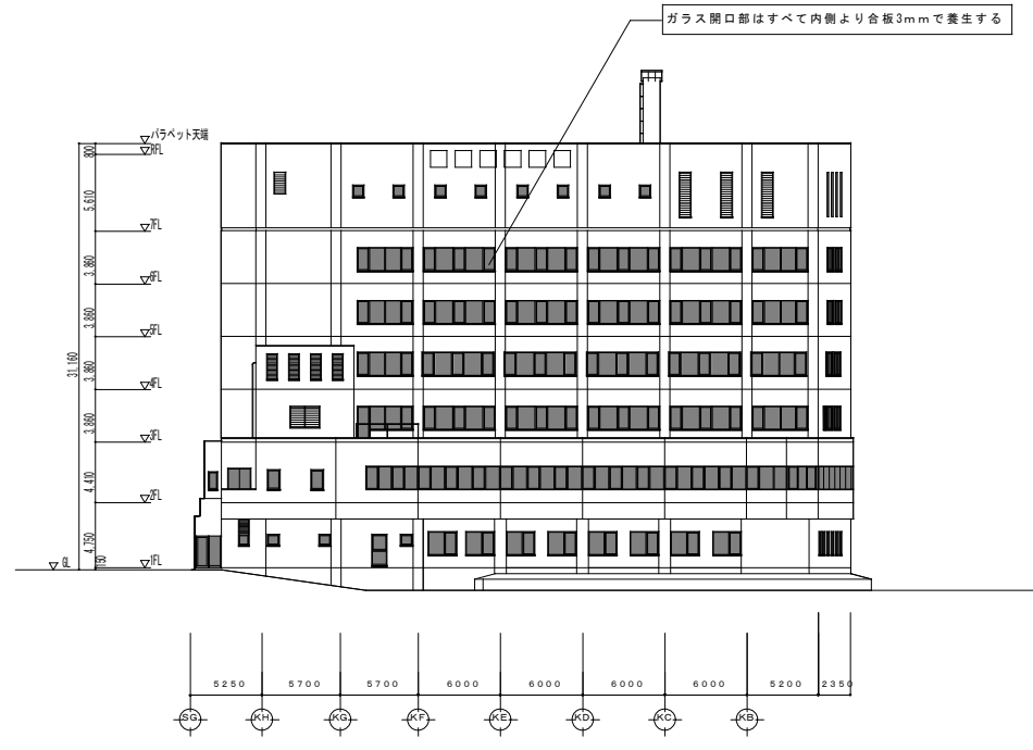
管理棟西立面図
